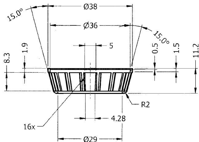
SECTION D-D
