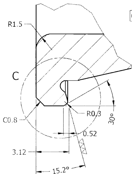
DETAIL B ( 5 : 1 )
