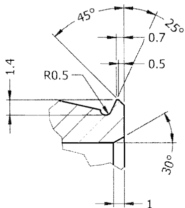
DETAIL A ( 3 : 1 )
